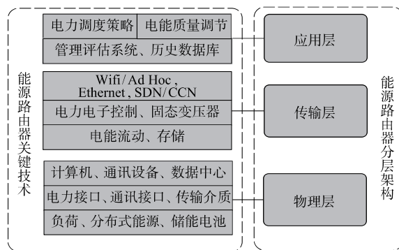
图6 能源路由器结构
