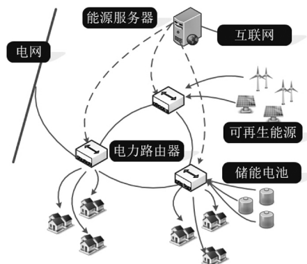
图2 日本数字电网框架模型
