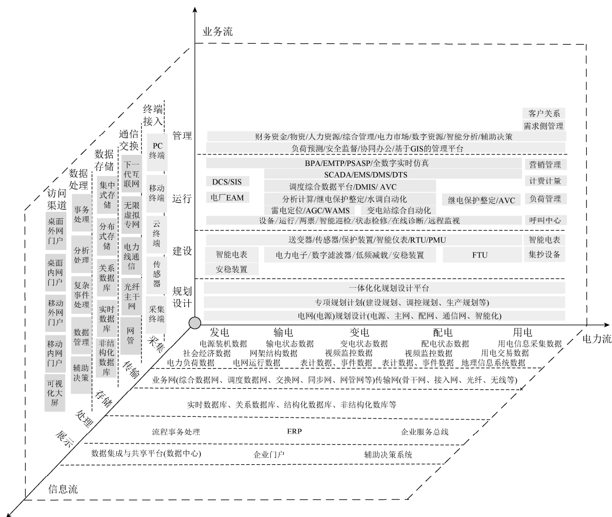
图2 能源互联网中的“三流合一” Fig. 2 “Fusion of triple flows” in energy internet
