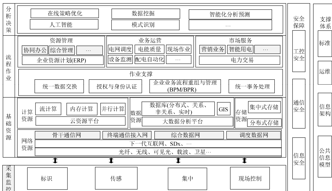
图3 能源互联网信息通信体系结构
