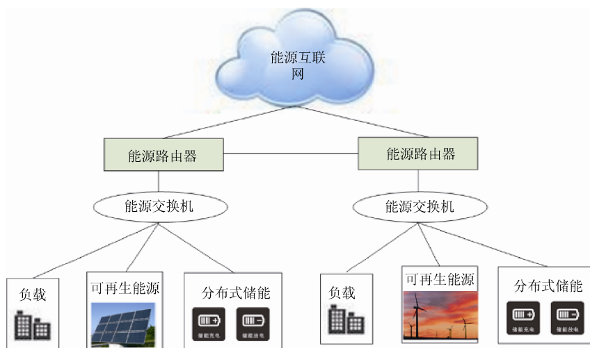
图 5 能源互联网组网示意图
